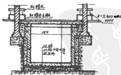
60平方米房间开挖及支撑剖面图
