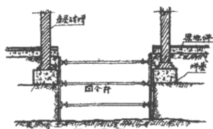
开挖时支撑示意图
